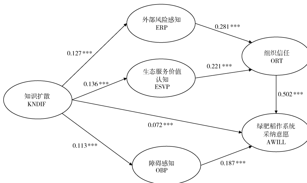
图 3 知识扩散影响农户绿肥稻作系统采纳意愿的部分中介效应结构模型
